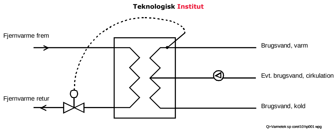
Fig. 17: Brugsvandsvarmeveksler med evt. brugsvandscirkulation.
