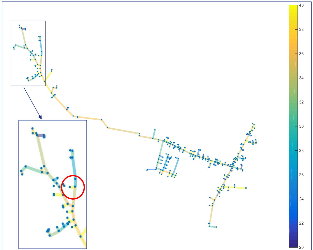
Figur 13: Beregnet returvandstemperatur i Hvam – Gl. Hvam baseret på målinger hos alle forbrugere i perioden 2. til 13. januar 2017.
